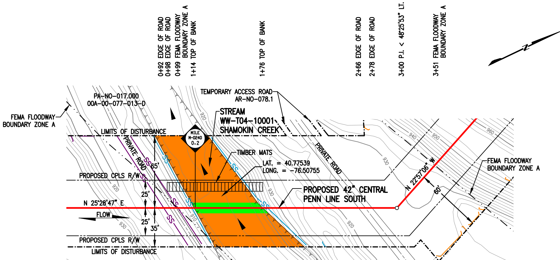
PLAN SCALE: 1" = 50'
